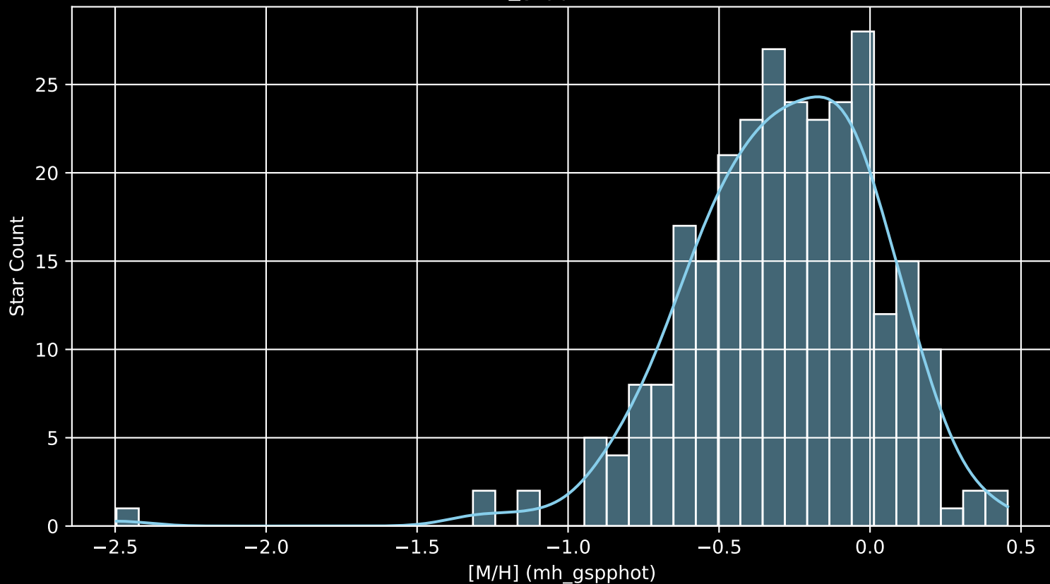
GALAH DR4 Field: [276] [M/H] (mh_gspphot) (n= 274)
