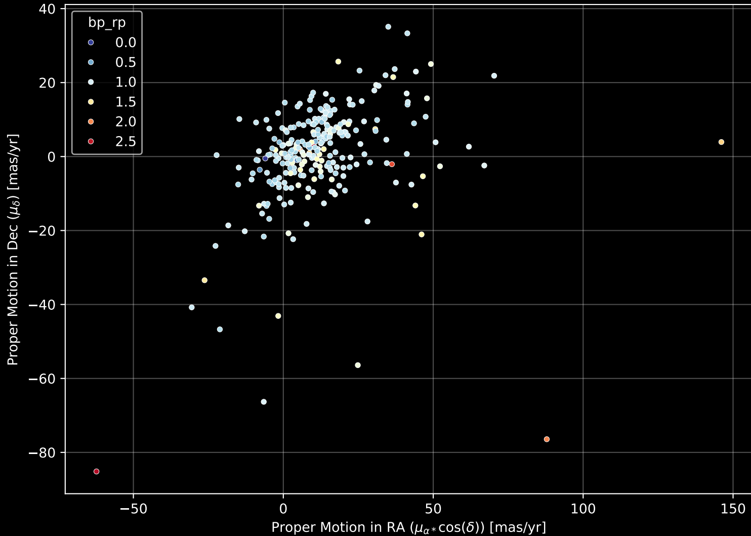
GALAH DR4 Field: [276] Proper Motion Diagram (n= 274)
