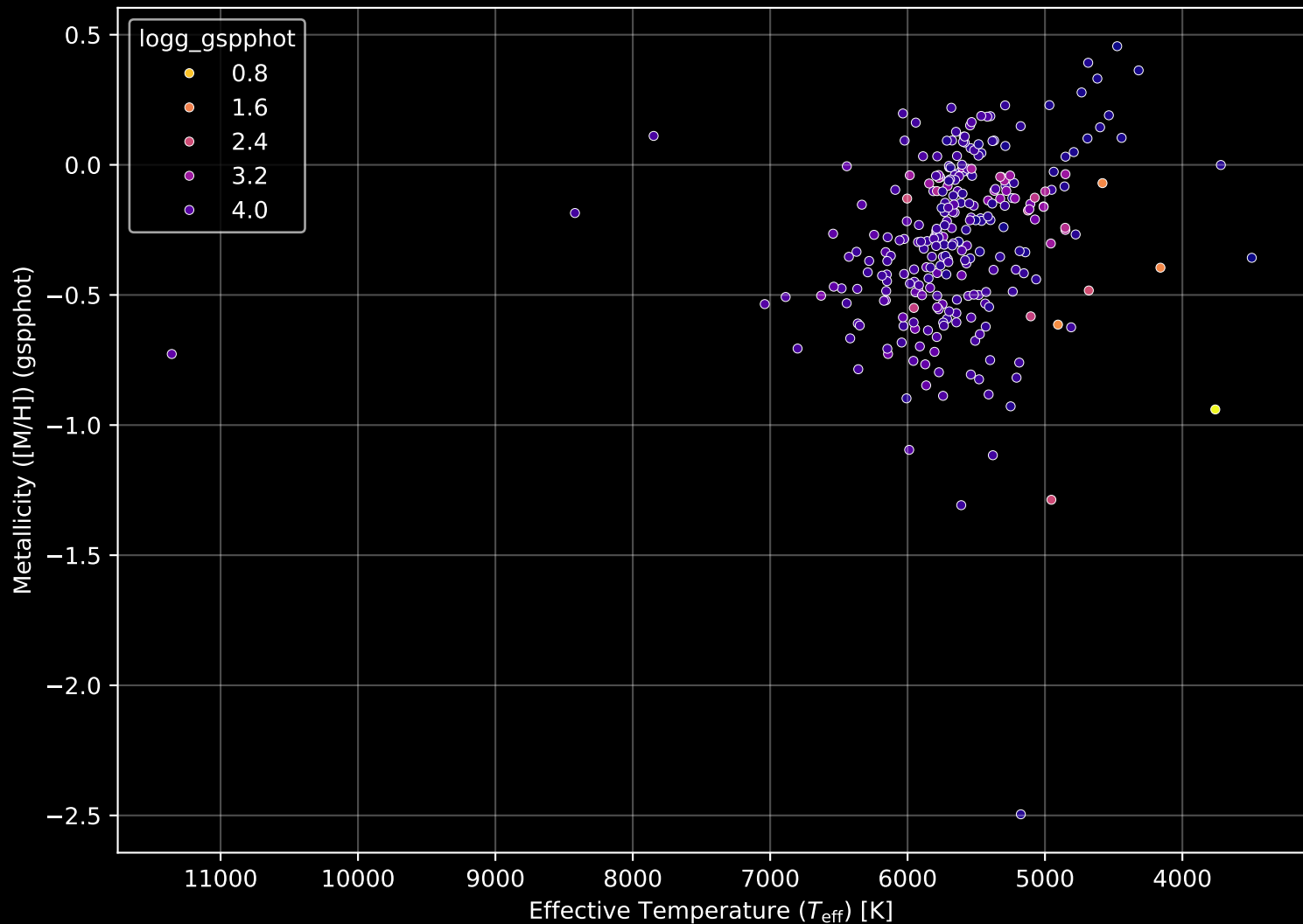
GALAH DR4 Field: [276] Stellar Population Parameters (n= 274)
