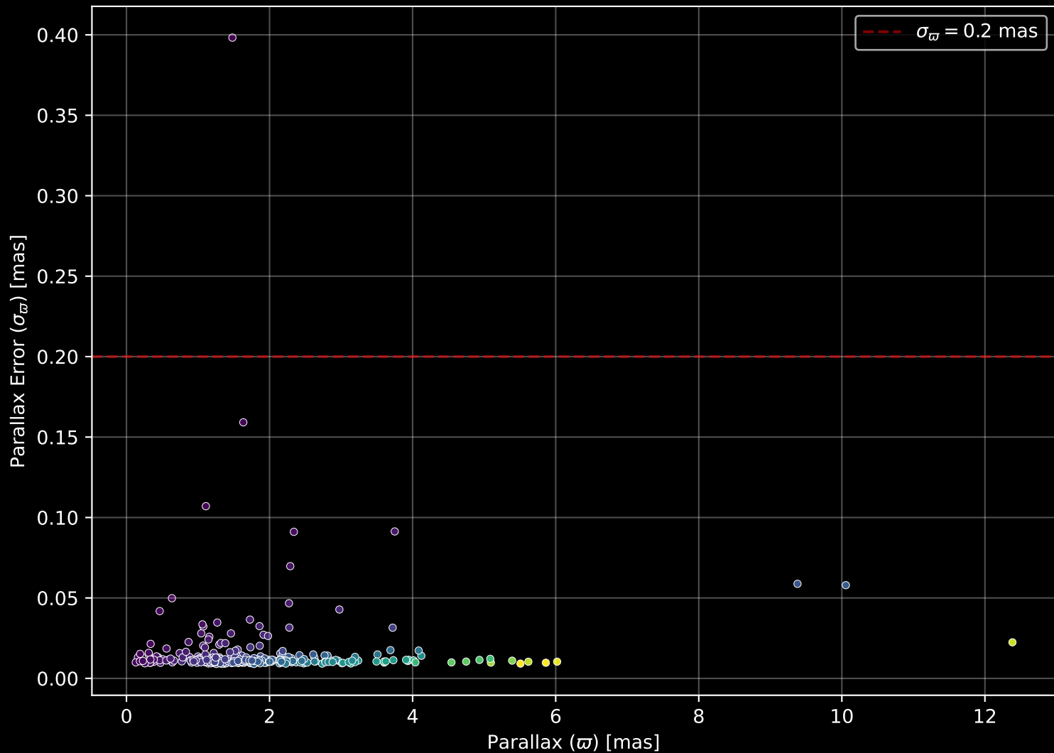
GALAH DR4 Field: [276] Parallax Quality (n= 274)
